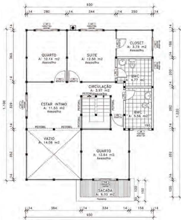
PAVIMENTO SUPERIOR 488,39 m 2
