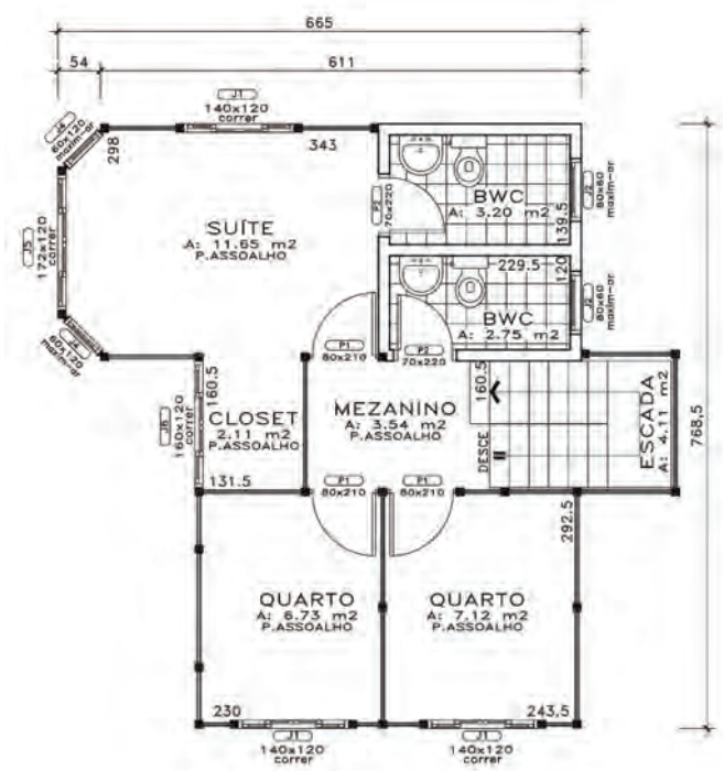
PAV. SUPERIOR A: 45,14 m 2
