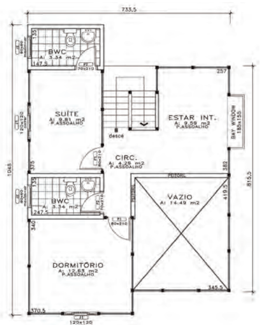
PAVIMENTO SUPERIOR A: 52,64 m 2
