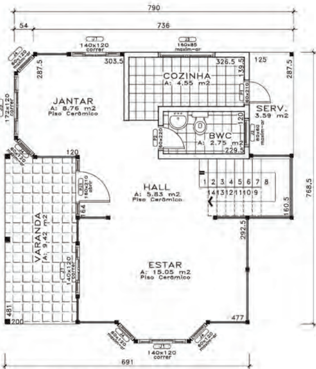
PAV. TERREO A: 59,15 m 2
