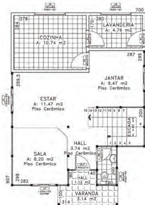
PISO TERREO A: 63.72 m 2
