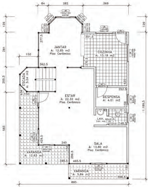
PAV. TÉRREO A: 99.36 m 2
