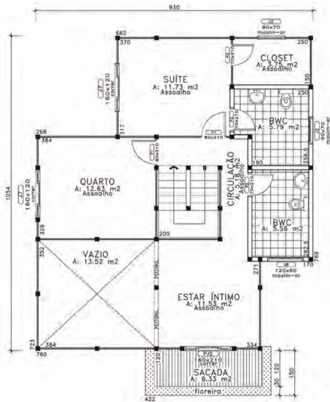
PAVIMENTO SUPERIOR A: 77.58 m 2
