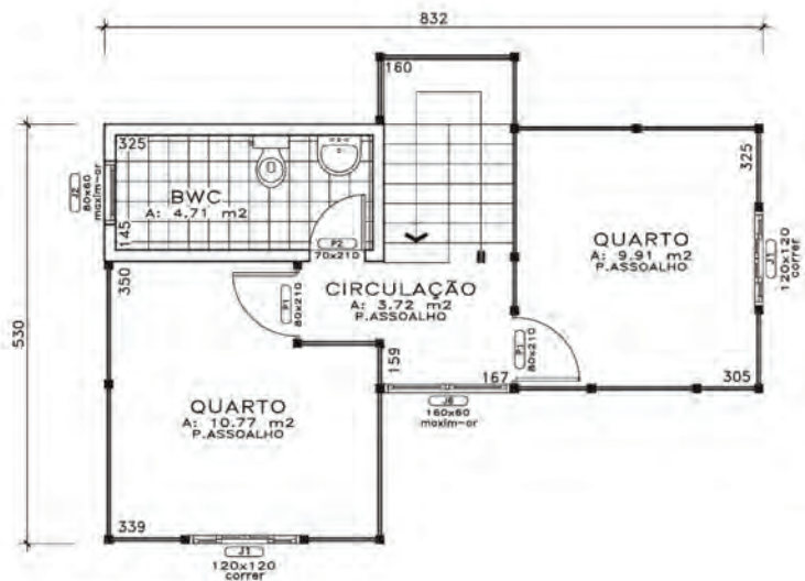
PAV. SUPERIOR A: 36.59 m 2
