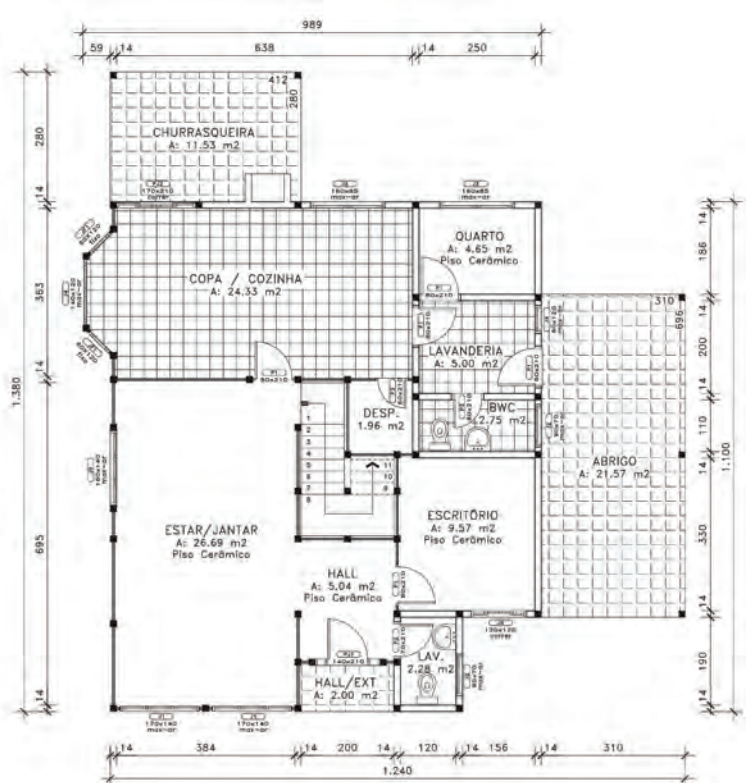
PAVIMENTO TÉRREO 133,28 m 2
