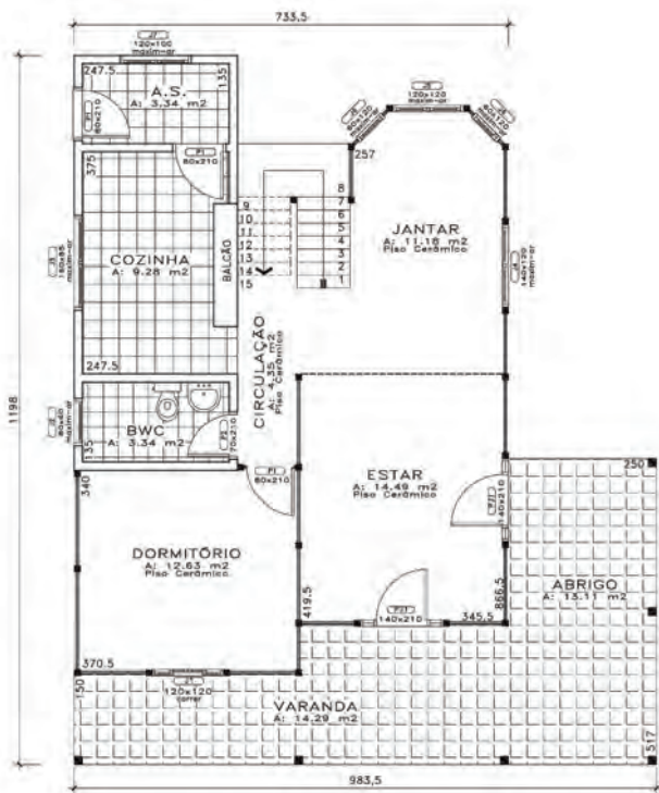
PAVIMENTO TERREO A: 95,31 m 2
