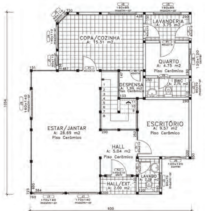
PAVIMENTO TERREO A: 89.38 m 2
