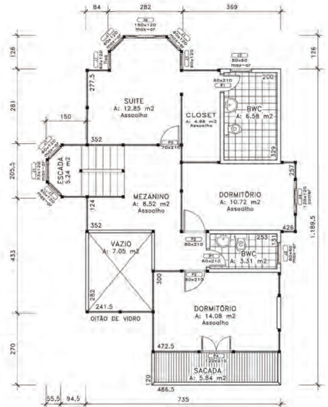
PAV. SUPERIOR A: 81.33 m 2
