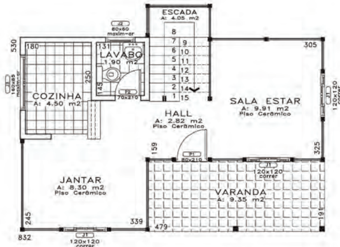
PAV. TERREO A: 45.73 m 2
