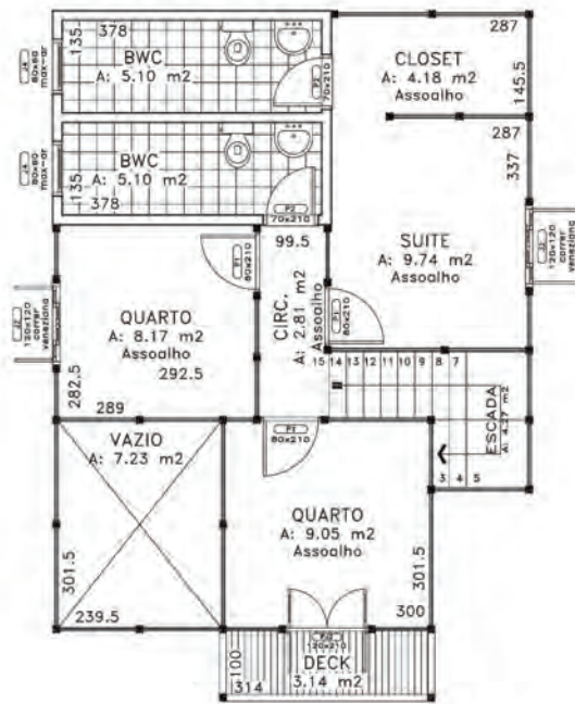
PISO SUPERIOR A: 56.49 m 2
